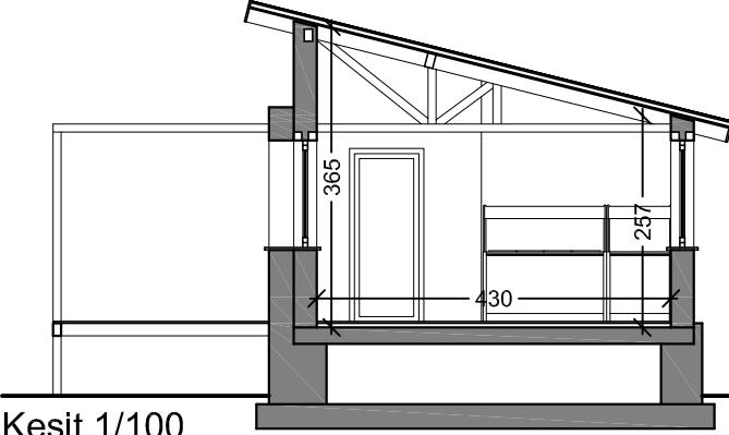
Kesit 1/100
